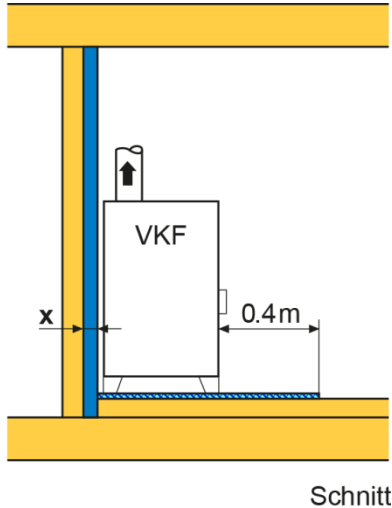
Schnitt
