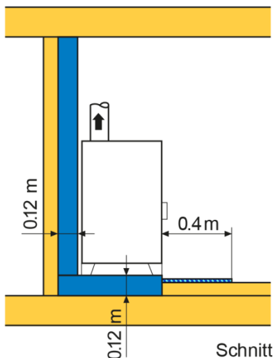
Schnitt
